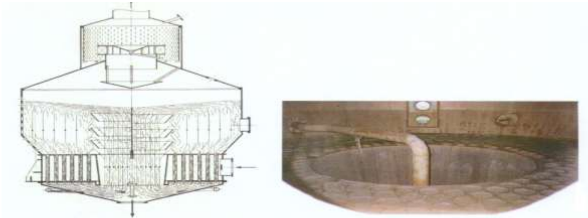
Foto 13: Cozedor batelada, vertical com calandra fixa e plana e sua vista interna
